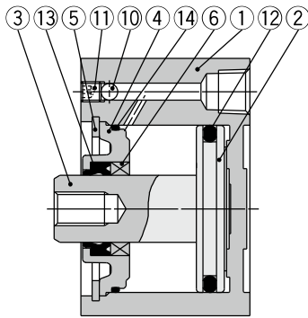
A-A section (Port on rod end)
